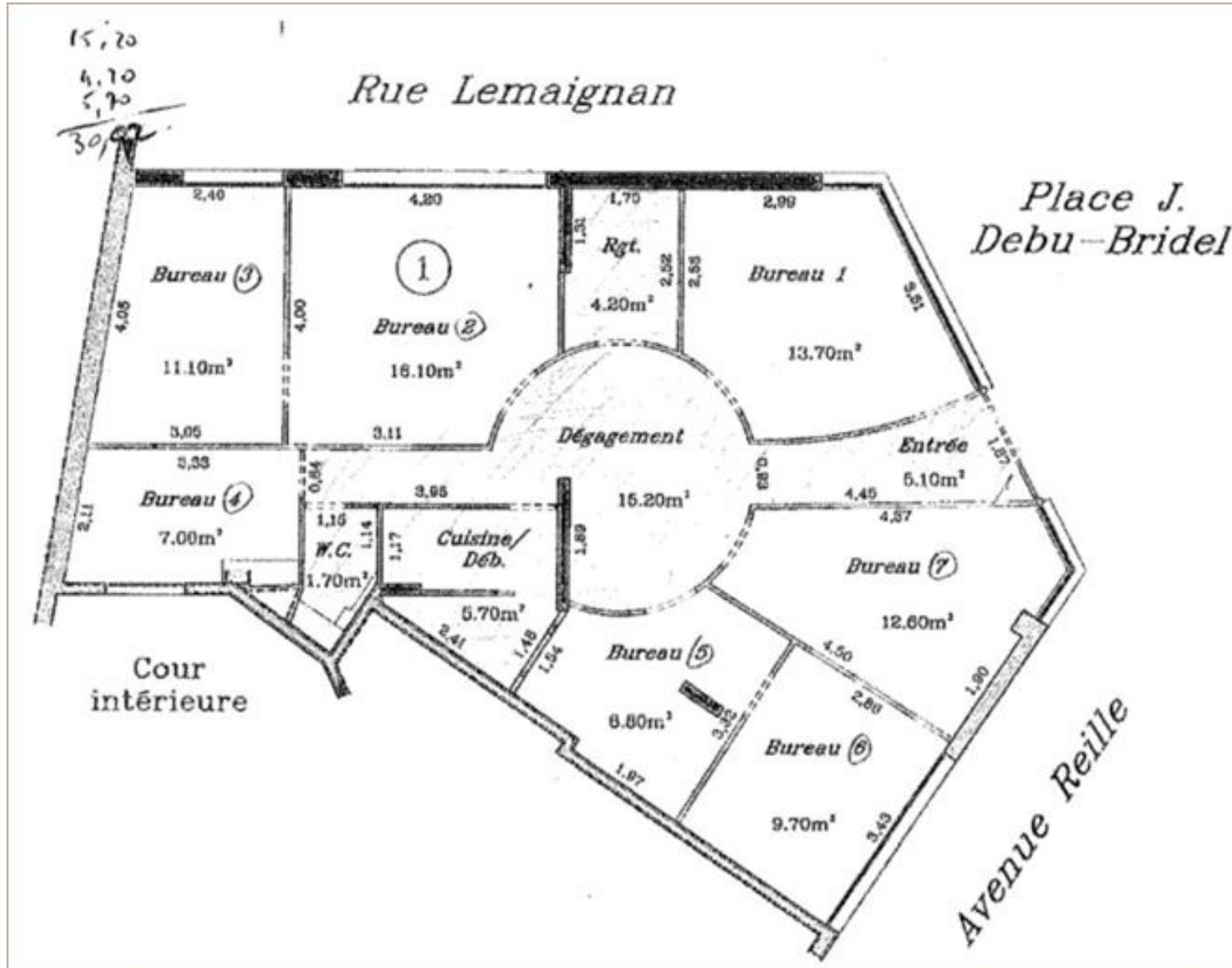
Plan rdc
