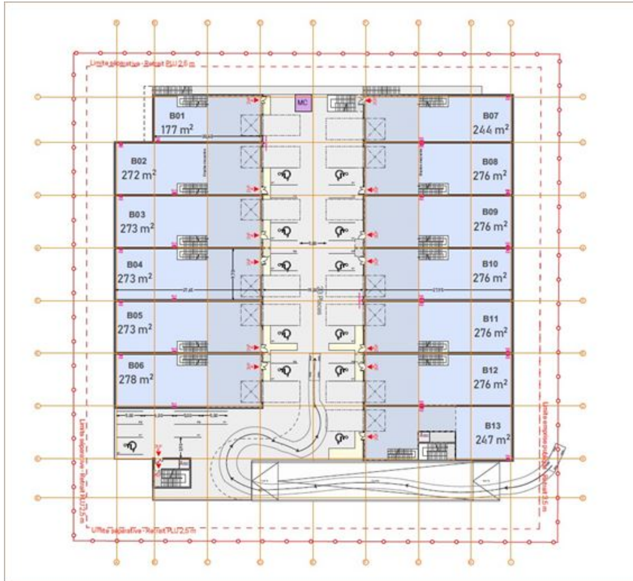
Plan r+2
