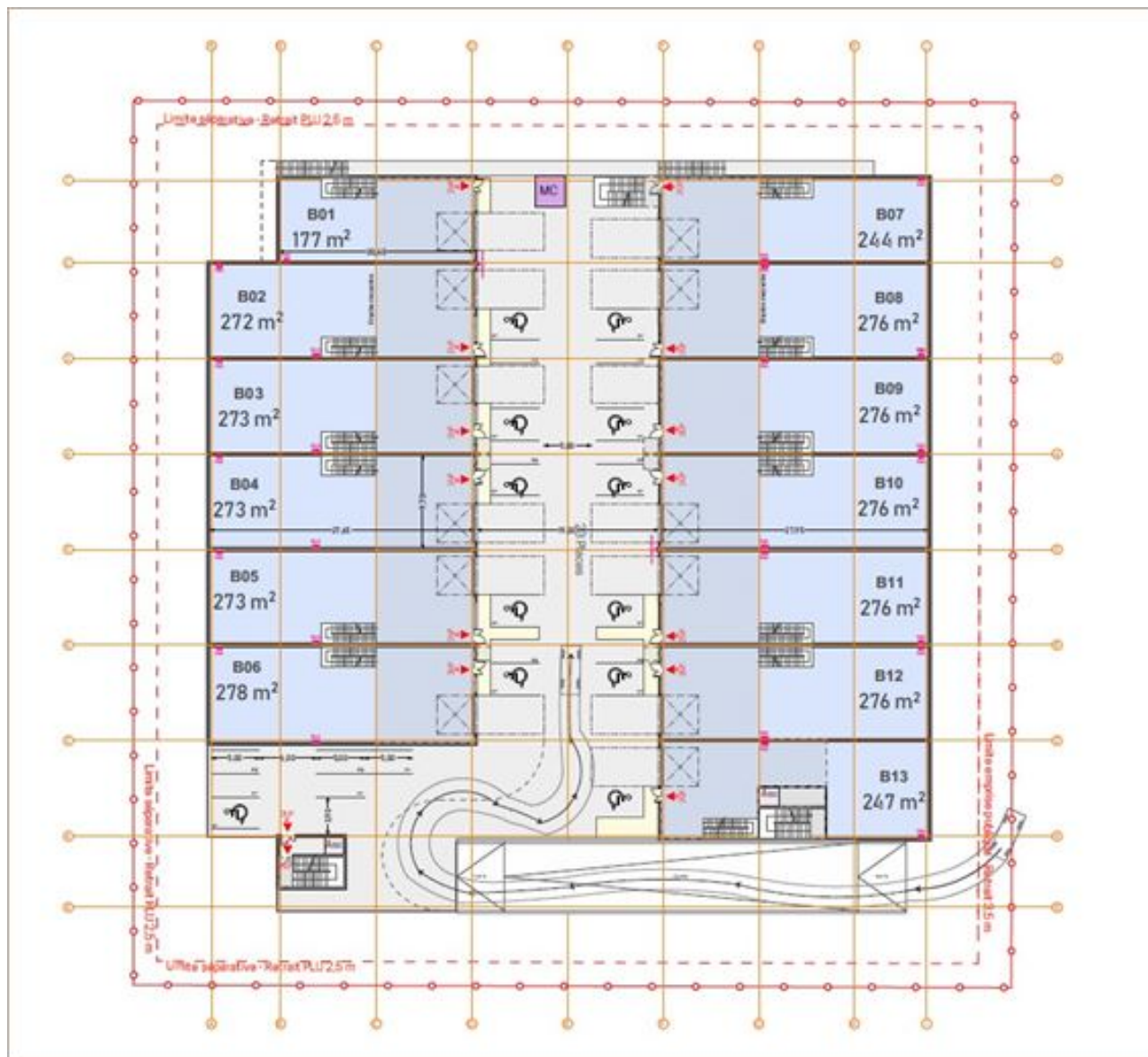
Plan r+2
