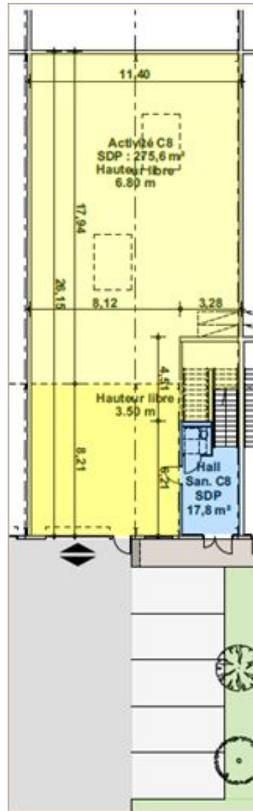
Plan rdc
