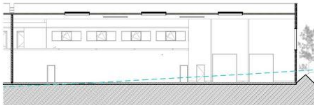
Bât B.02 - Coupe AA
