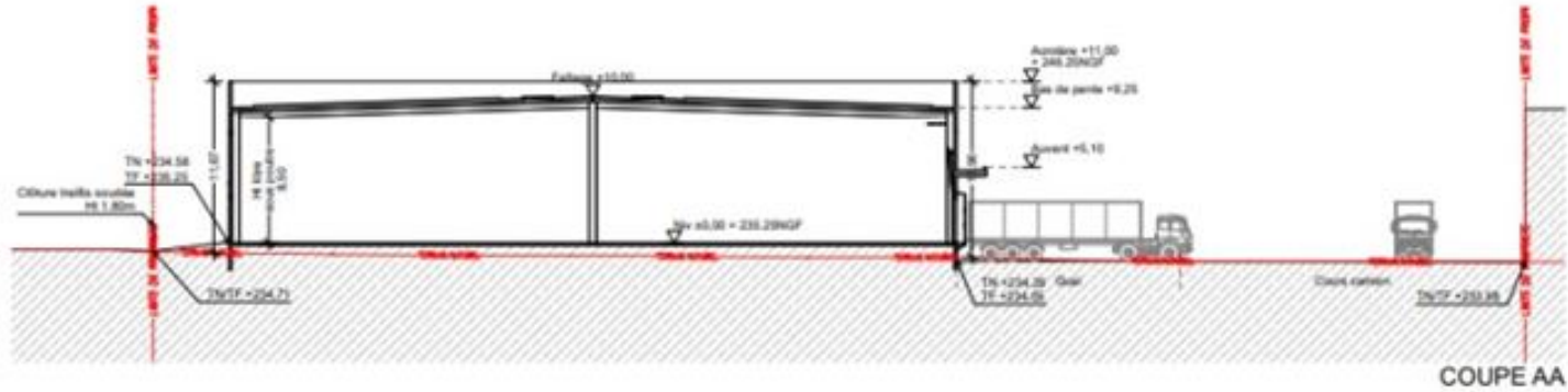
COUPE AA
